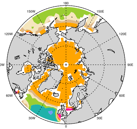
ESMF_regrid (conserve)
