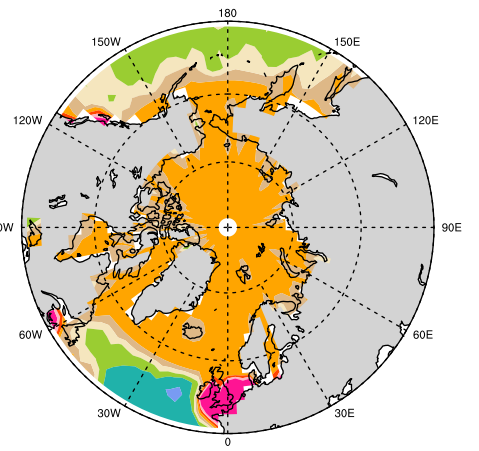
ESMF_regrid (conserve)
