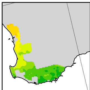
(b) ERA-Interim
