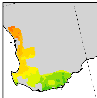
(d) CSIRO
