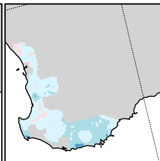
(h) CSIRO bias
