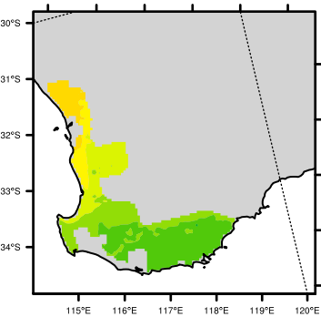
(b) ERA-Interim
